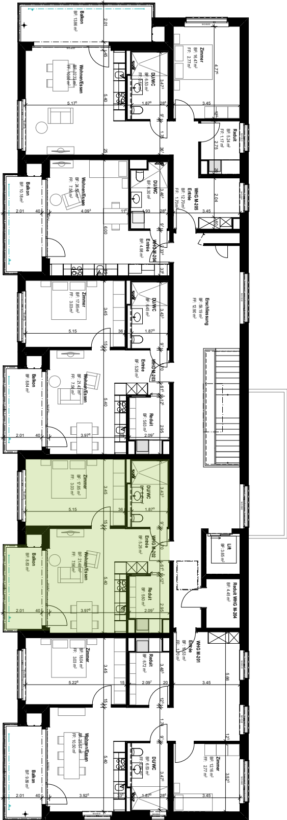
Haus M 2. Obergeschoss 2.5 Zimmer Wohnung M-202 Nutzfläche: 56.4 m 2 ohne Balkon
