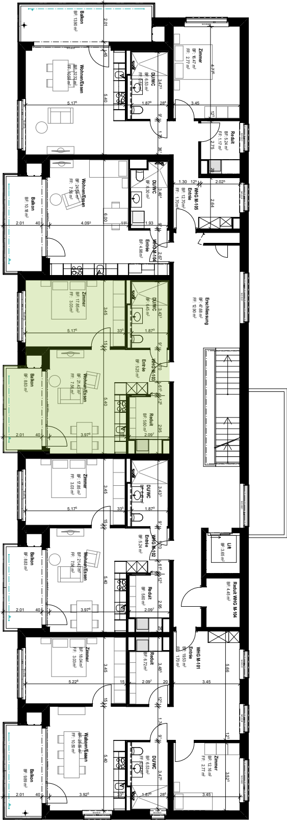
Haus M 1. Obergeschoss 2.5 Zimmer Wohnung M-103 Nutzfläche: 56.4 m 2 ohne Balkon
