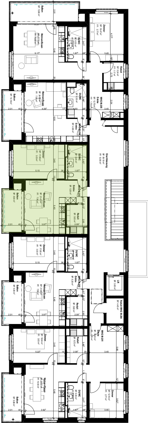
Haus M 2. Obergeschoss 2.5 Zimmer Wohnung M-203 Nutzfläche: 56.4 m 2 ohne Balkon
